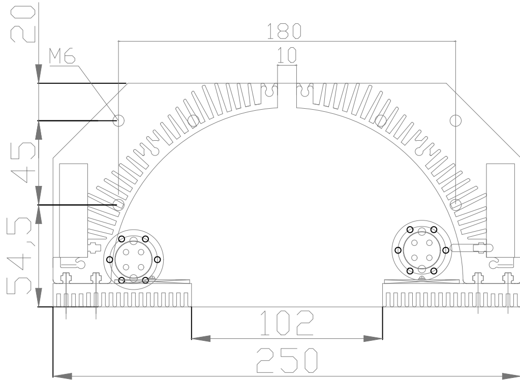
LDM隧道光源尺寸示意图
